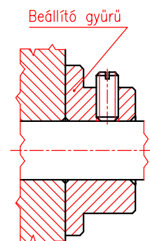
Axiális beállítás (pl. szereléskor)
